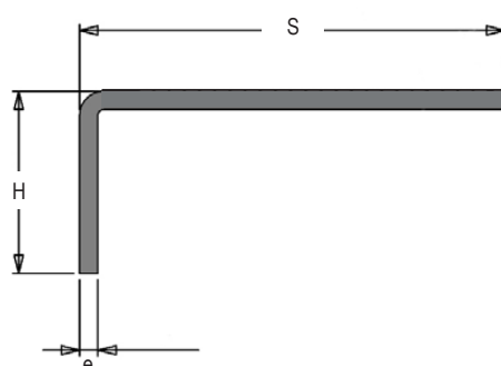
NDM VDi arabesque avec perçage / NDM VDi arabesque with drilling
