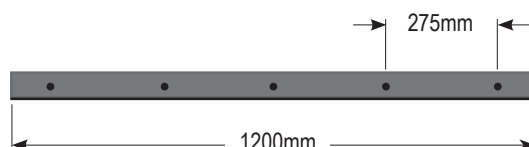
NDM VDi strié avec perçage / NDM VDi striped with drilling
